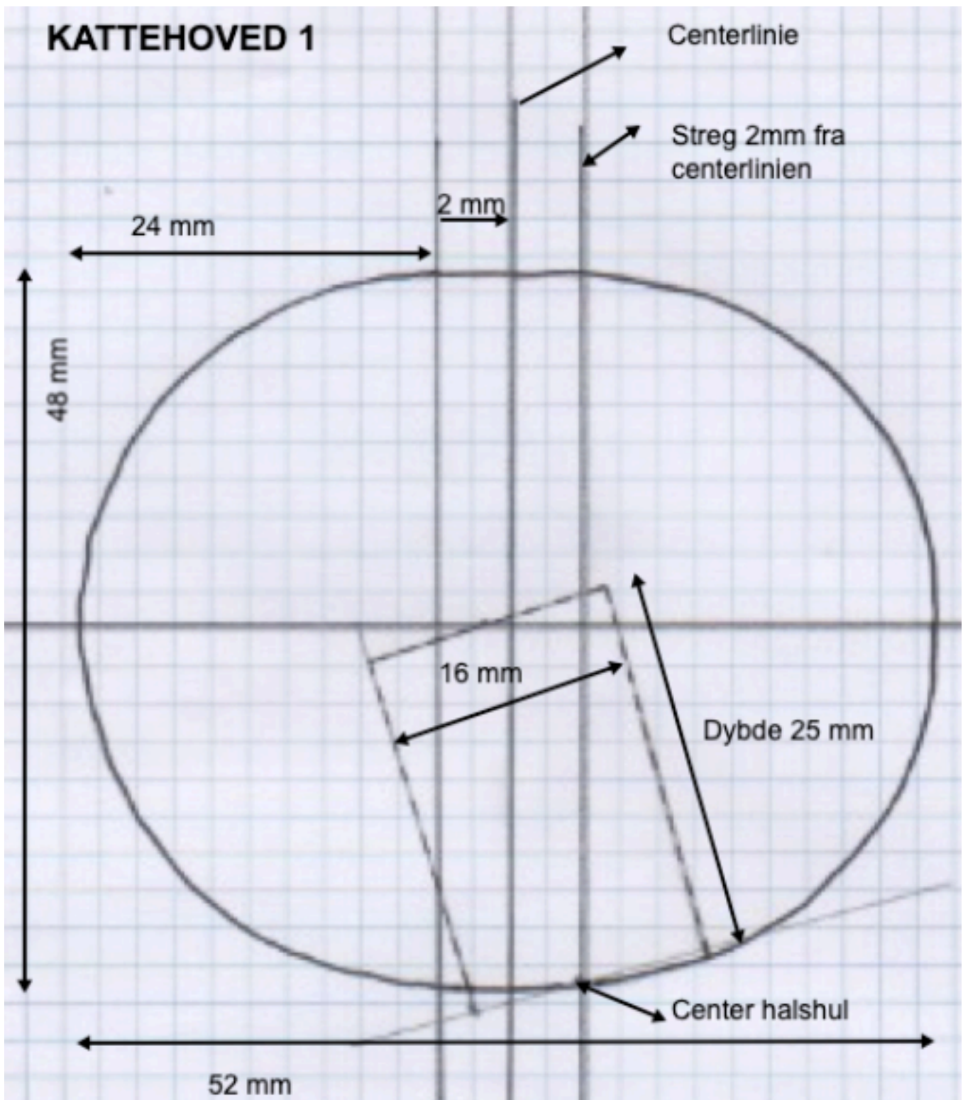
Detailtegning hovedet-1
